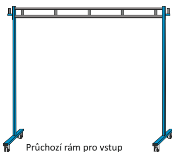
Průchozí rám pro vstup do vzniklého svařovacího boxu.
