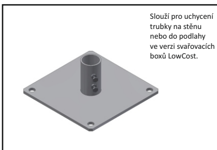
Patka trubky obj. č.: WZ-ROHRBE-STI-2
