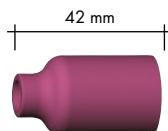
Standardní provedení
